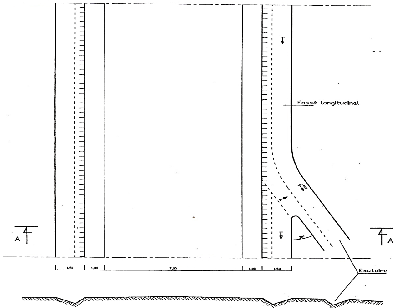
COUPE A-A
